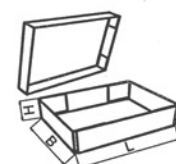
FEFCO 0307
