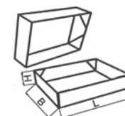
FEFCO 0309
