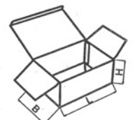
FEFCO 0216
