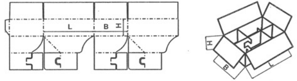
FEFCO 0718
