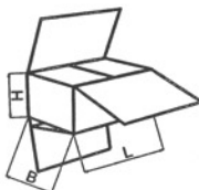
FEFCO 0207
