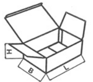
FEFCO 0212
