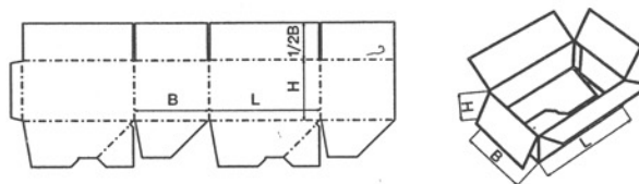
FEFCO 0712
