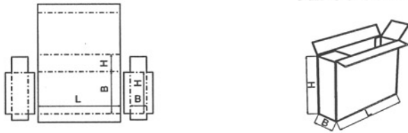
FEFCO 0700
