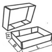
FEFCO 0301
