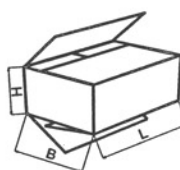
FEFCO 0206
