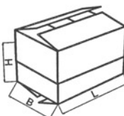
FEFCO 0321
