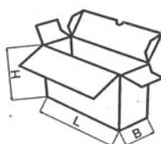
FEFCO 0230
