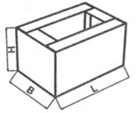
FEFCO 0210
