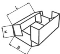
FEFCO 0415
