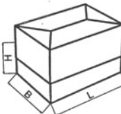
FEFCO 0323
