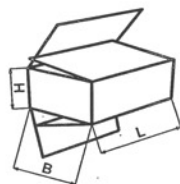
FEFCO 0204
