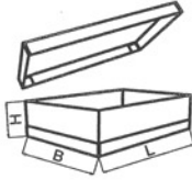
FEFCO 0311
